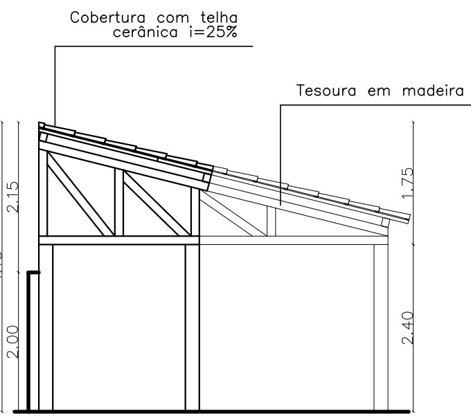
VISTA B - ESTACIONAMENTO ESCALA 1:75
