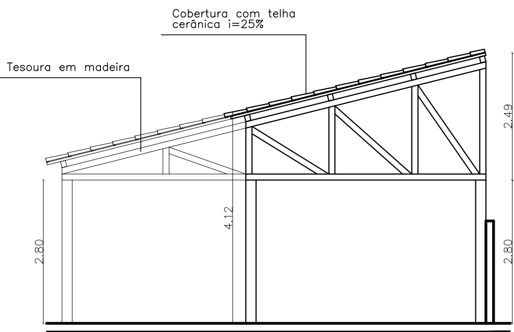
VISTA A - MULTIUSO ESCALA 1:75
