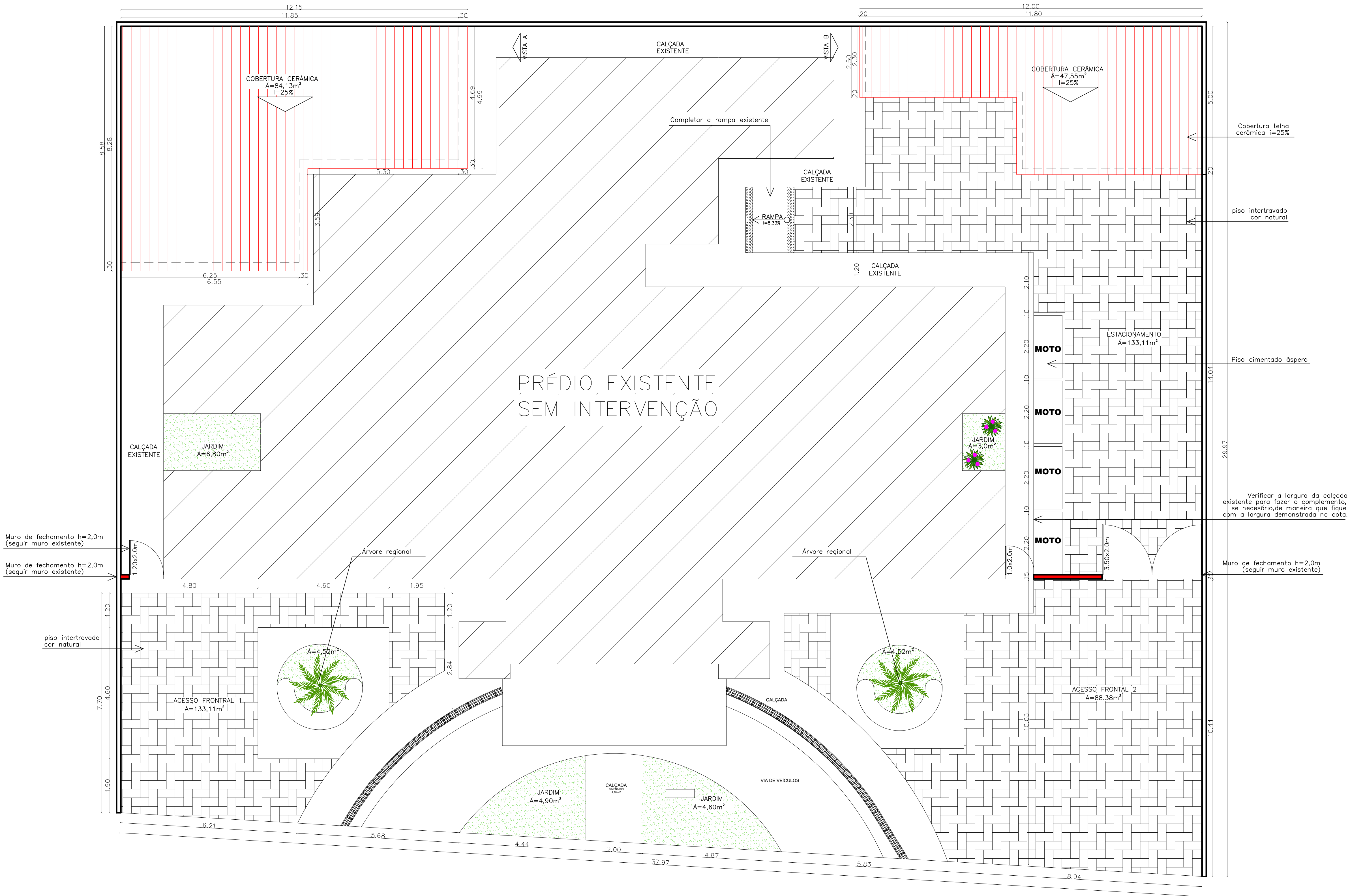
PLANTA DE COBERTURA ESCALA 1:75
